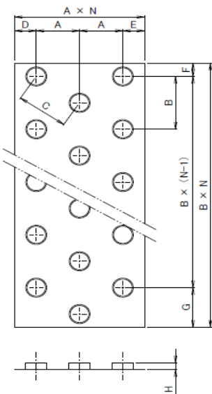
＜千鳥配列＞
