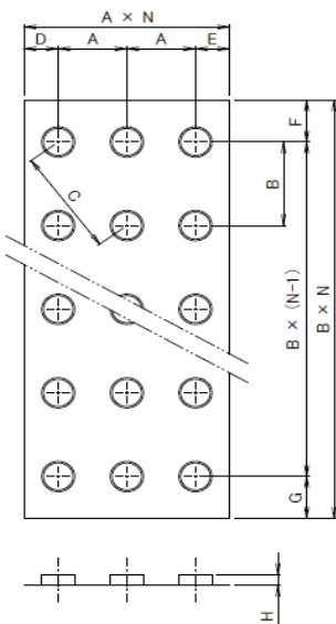
＜並列配列＞
